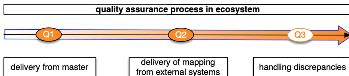
Abbildung 4: QS – Prozess
