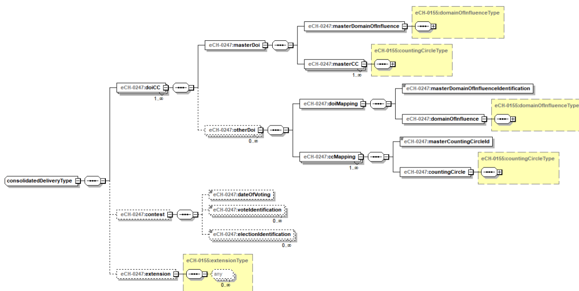
Abbildung 7: consolidatedDelivery
