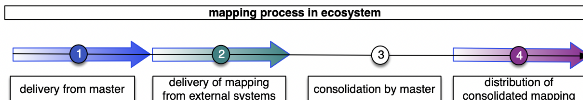
Abbildung 3: Mapping-Prozess
