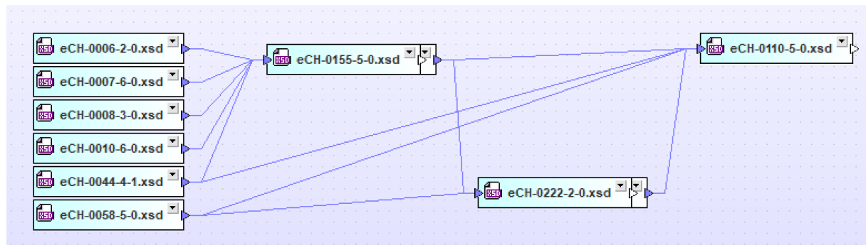
Abbildung 20: Abhängigkeiten
