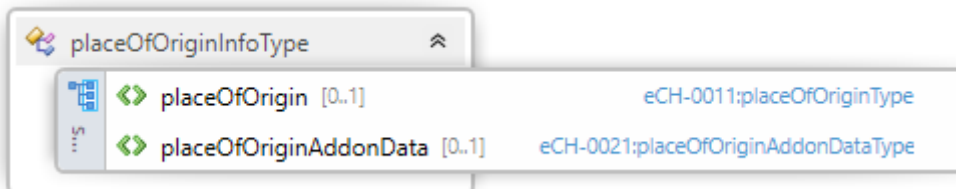
Abbildung 23: placeOfOriginInfoType
