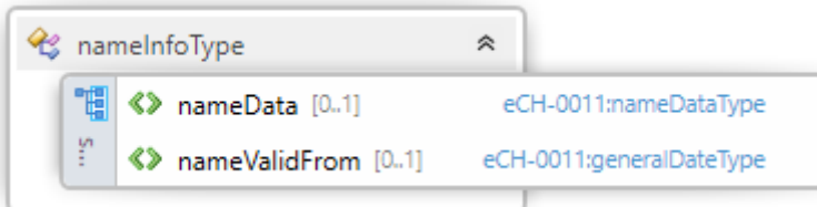
Abbildung 20: nameInfoType
