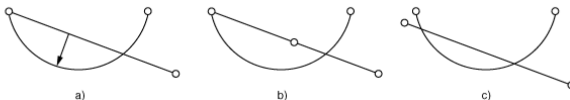
Figure 15 : a) La flèche ne doit pas excéder la tolérance indiquée ; b), c) recouvrements non permis pour une polyligne, le segment de droite et l'arc de cercle en intersection n'ayant pas leur origine en un point d'appui commun.
