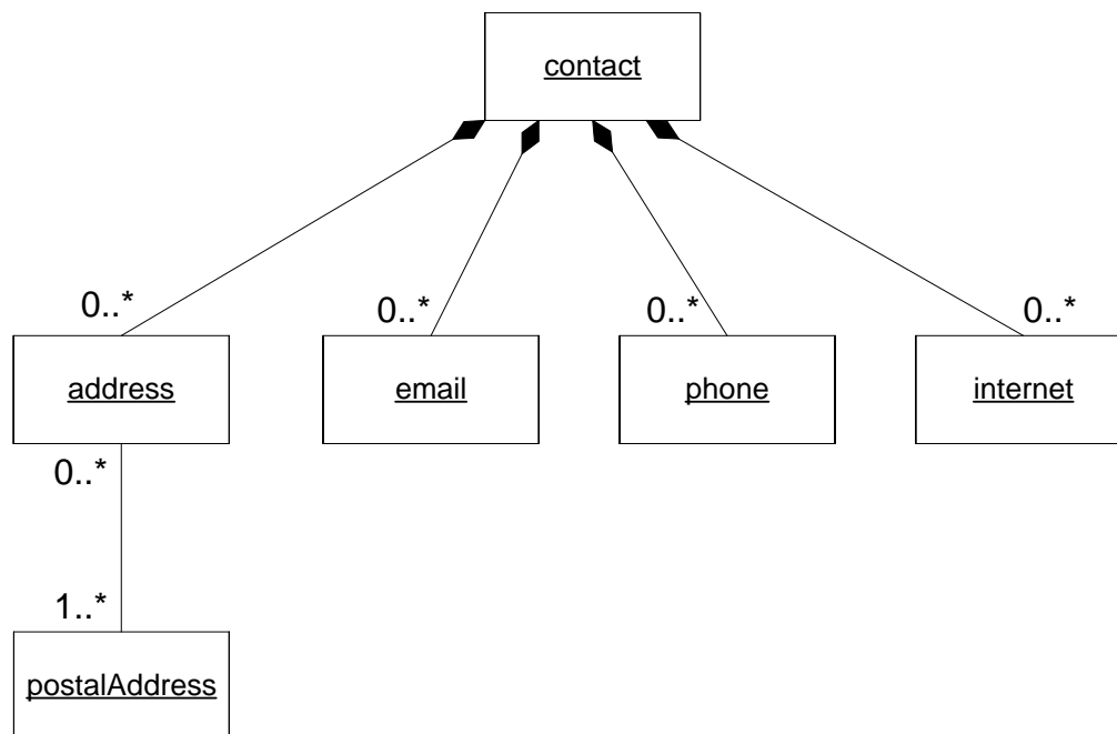
Figure 1 : modèle de donnée pour contact
