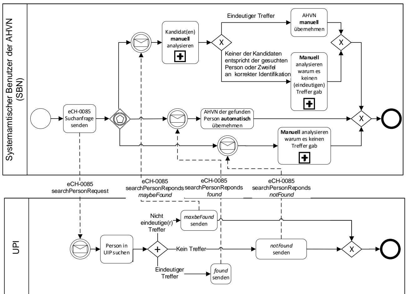
Abbildung 9: Prozessbeschreibung der Suche der AHVN einer bestimmten Person
