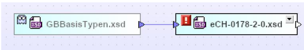
Abbildung 8: Abhängigkeiten
