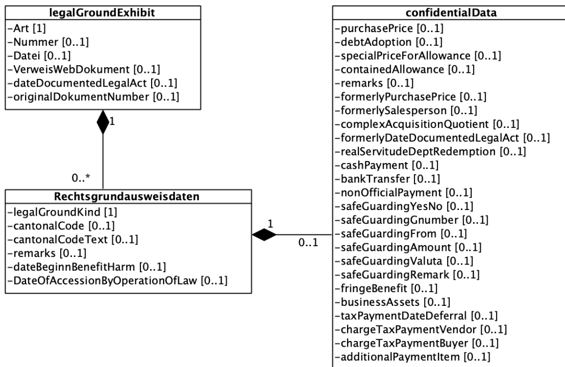
Abbildung 3: Austauschdatenmodell
