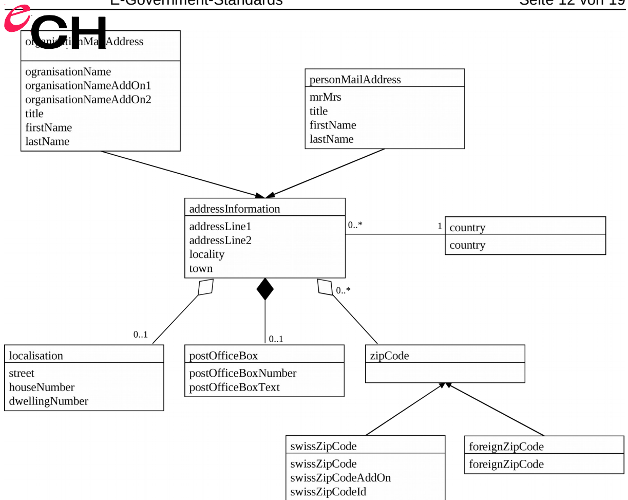
Abbildung 1: UML-Diagramm zur Postadresse
