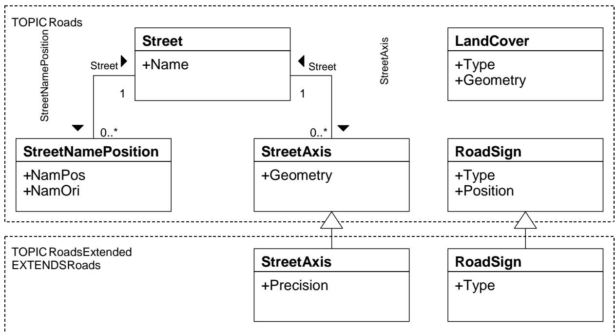
Abbildung 26: UML-Klassendiagramm der Datenmodelle.
