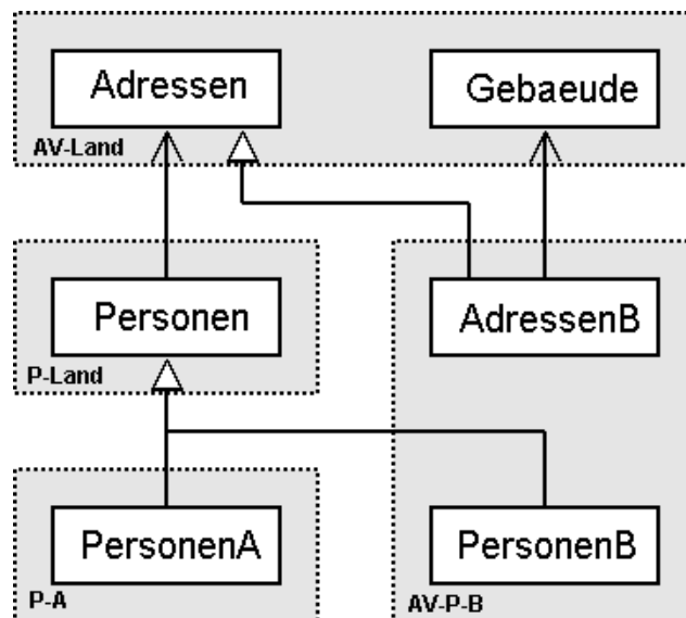
Abbildung 3: Vererbungs-Hierarchie von Adresse, Person und Gebäude.
