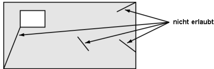
Abbildung 23:Nicht erlaubte Linien von Flächen.
