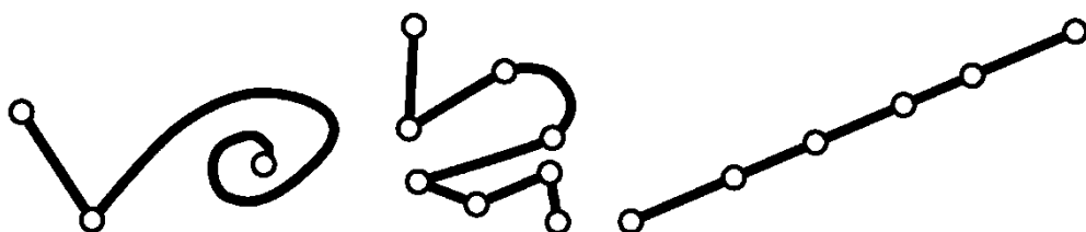
Abbildung 14: Beispiele von (ebenen) einfachen Linienzügen.
