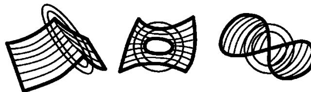
Abbildung 17: Beispiele von Punktmengen im Raum, die nicht Flächenelemente sind (ein doppelter Kreis bedeutet hier "nicht glatt").
