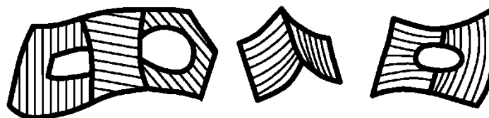
Abbildung 18: Beispiele von Flächen im Raum.
