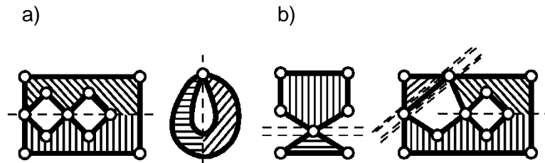
Abbildung 21: a) Beispiele von allgemeinen ebenen Flächen; b) Beispiele von ebenen Mengen, die nicht allgemeine Flächen sind, weil ihr Inneres nicht zusammenhängend ist. Diese ebenen Mengen können aber in allgemeine Flächen unterteilt werden ("---" zeigt die Unterteilung in Flächenelemente und "====" die Unterteilung in allgemeine Flächen).
