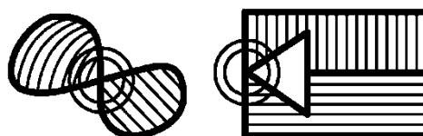
Abbildung 19: Beispiele ebener Punktmengen, die nicht Flächen sind (ein doppelter Kreis bedeutet "singulärer Punkt").
