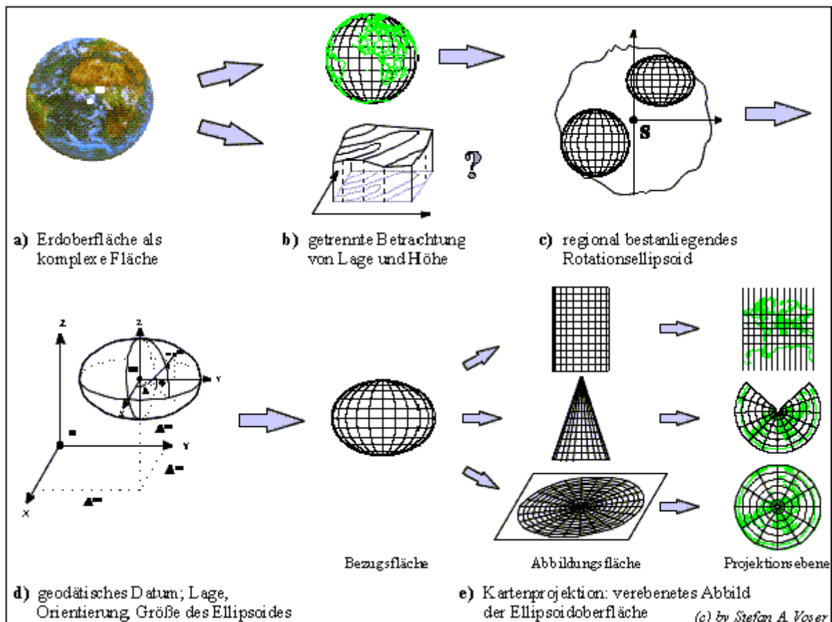
Abbildung I.1: Von der Erdoberfläche zu zweidimensionalen Lagekoordinaten.
