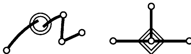
Abbildung 13: Beispiele von ebenen Mengen, die nicht Linienzüge sind (ein doppelter Kreis bedeutet hier "nicht stetig" und der Rhombus "nicht Bild eines Intervalls").
