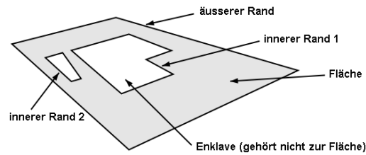
Abbildung 20: Ebene Fläche mit Rändern und Enklaven.
