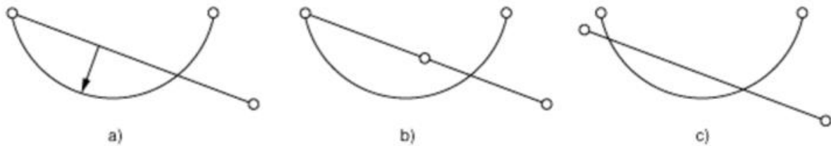
Abbildung 15: a) Die Pfeilhöhe darf nicht grösser als die angegebene Toleranz sein; b), c) unzulässige Überschneidungen eines Linienzuges, da Strecke und Kreisbogen, die sich treffen, nicht von einem gemeinsamen Stützpunkt ausgehen.
