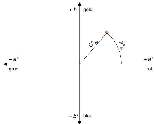
Abbildung H.4: Der Farbraum L*C* ab h* ab arbeitet mit polaren Koordinaten auf L*a*b*.
