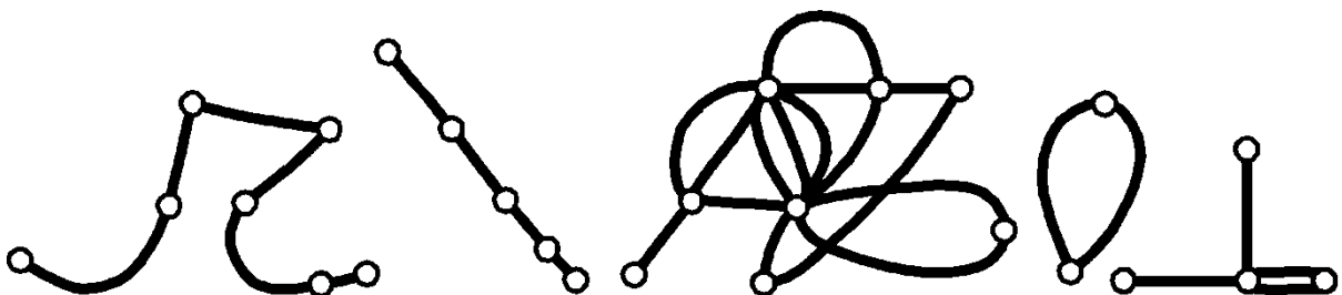
Abbildung 12: Beispiele von (ebenen) Linienzügen.
