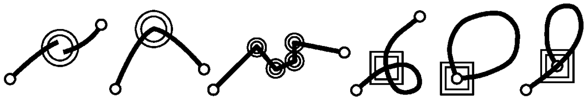
Abbildung 11: Beispiele von ebenen Mengen, die nicht Kurvenstücke sind (ein doppelter Kreis bedeutet "nicht glatt" und ein doppeltes Rechteck "nicht injektiv").
