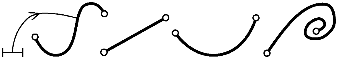
Abbildung 10: Beispiele von ebenen Kurvenstücken.
