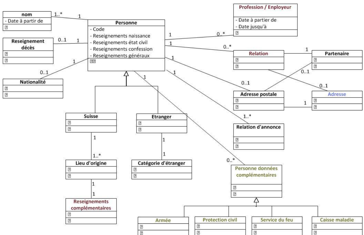
Figure 1: modèle de données concernant la personne
