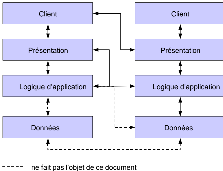
Figure 5-3 Voies de communication possibles
