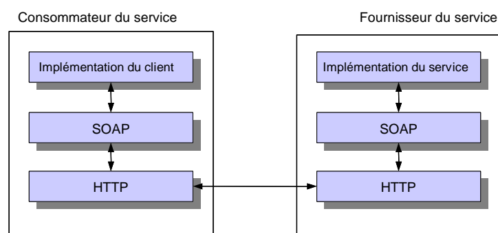
Figure 6-3 Pile de protocoles du message SOAP
