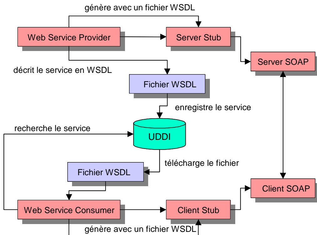
Figure 6-1 Dépendances des services en ligne
