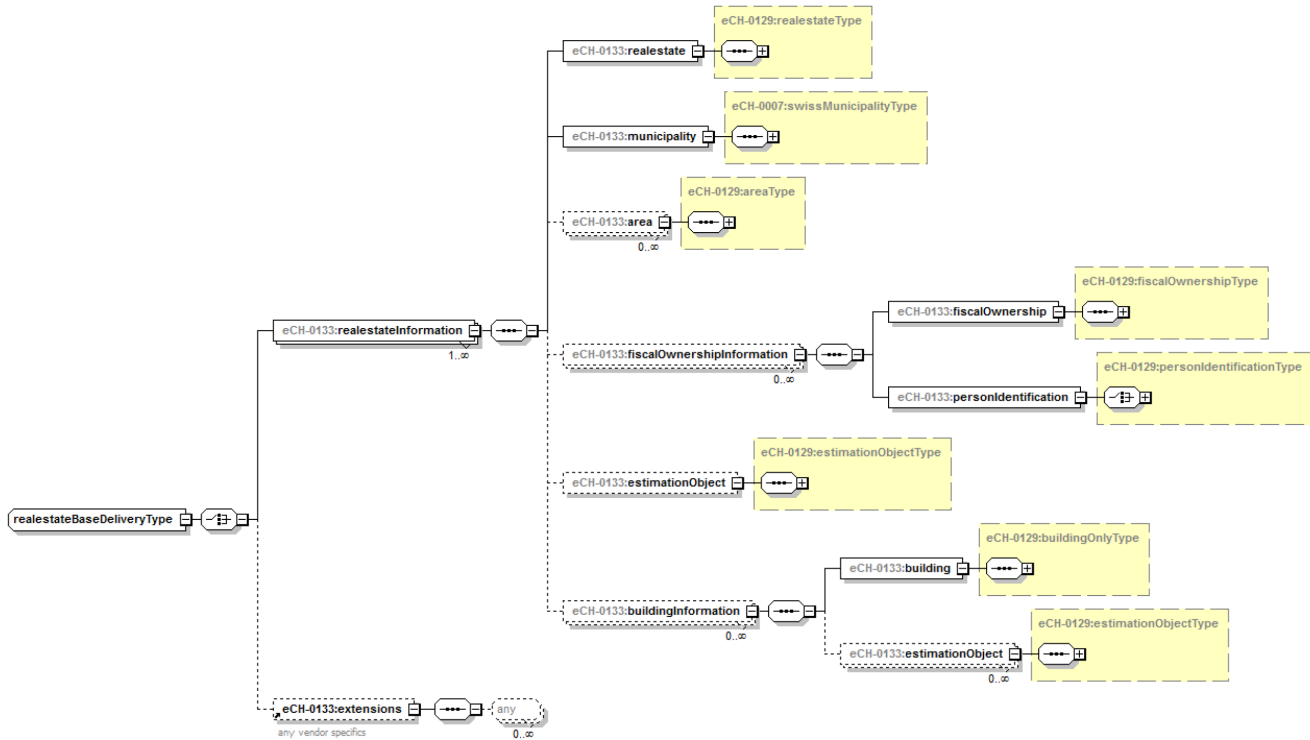
Abbildung 8: realestateBaseDelivery
