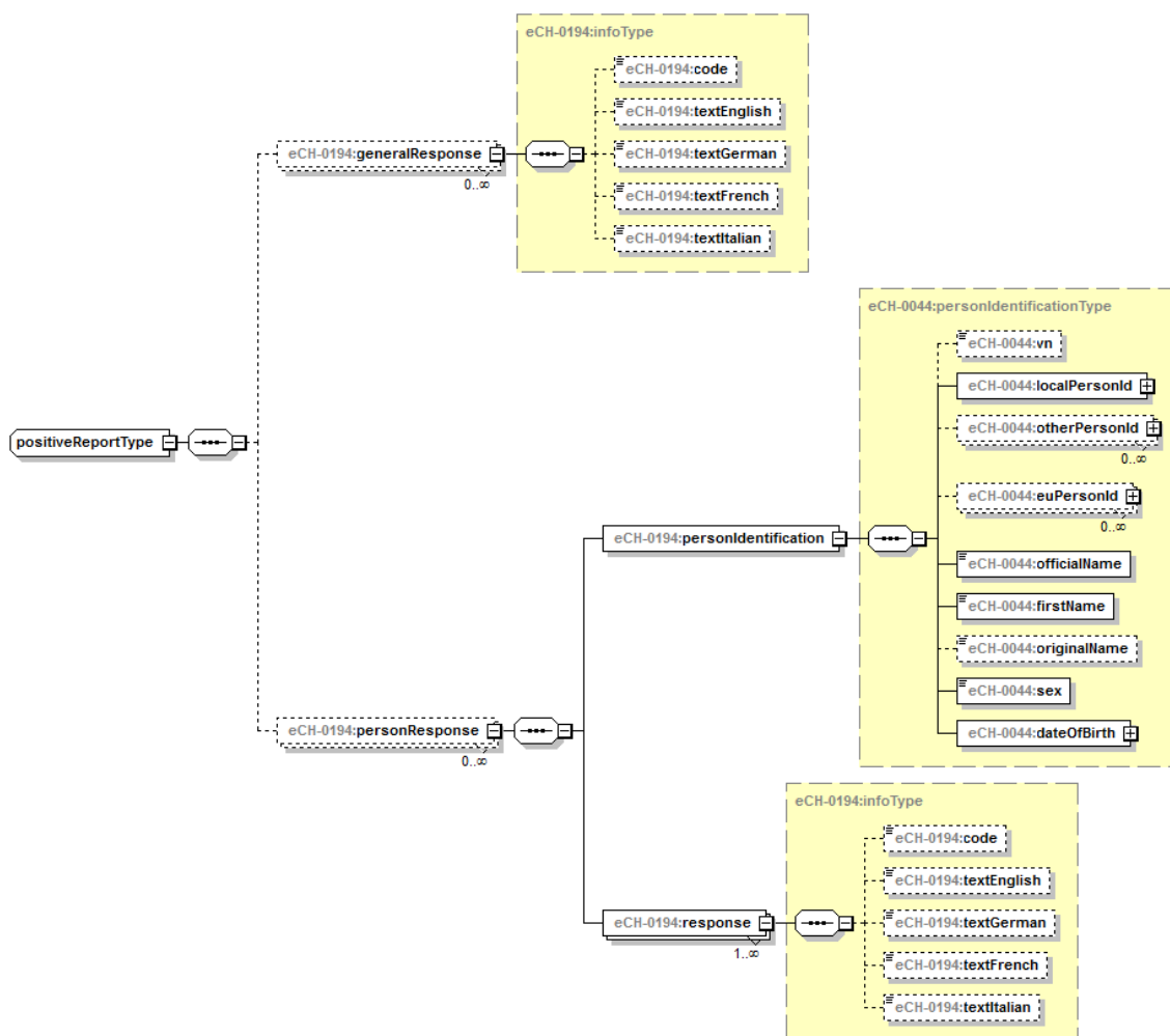
Abbildung 14: positiveReport
