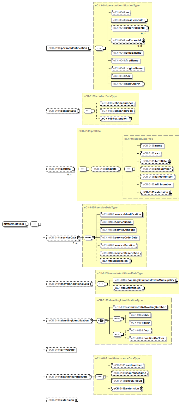
Abbildung 9: platformMoveIn
