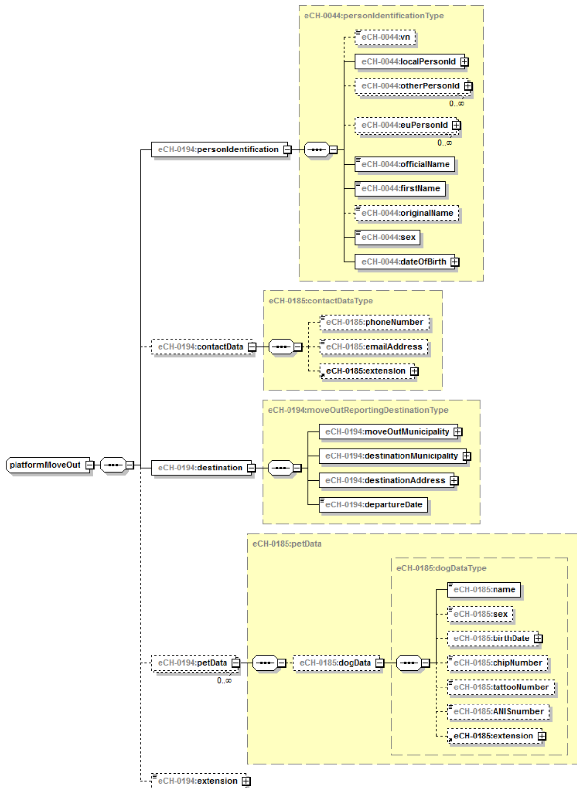
Abbildung 8: platformMoveOut
