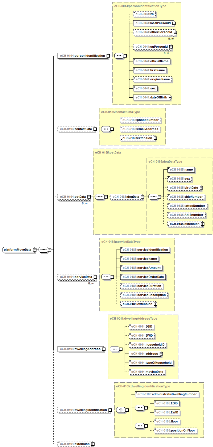
Abbildung 10: platformMoveData
