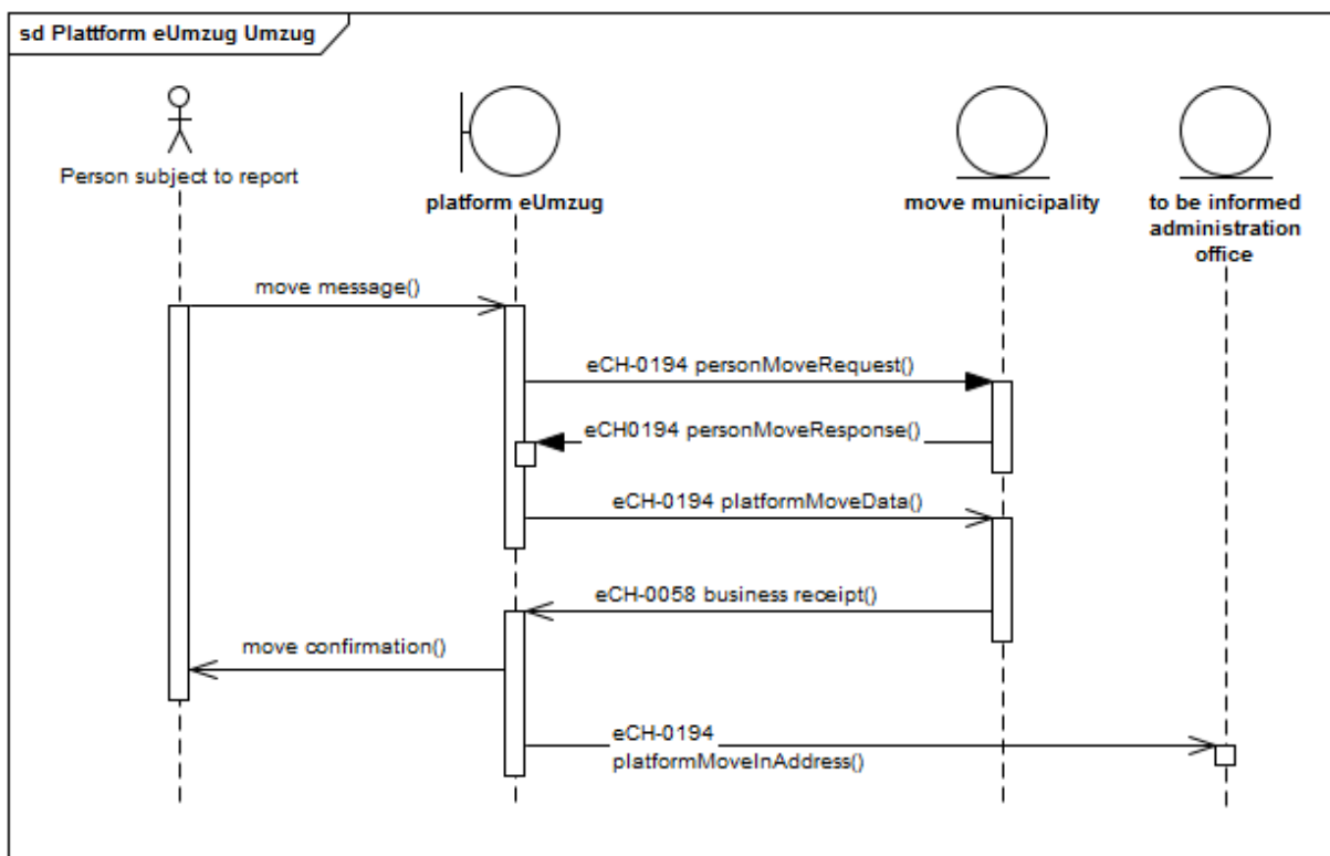
Abbildung 4: Umzug
