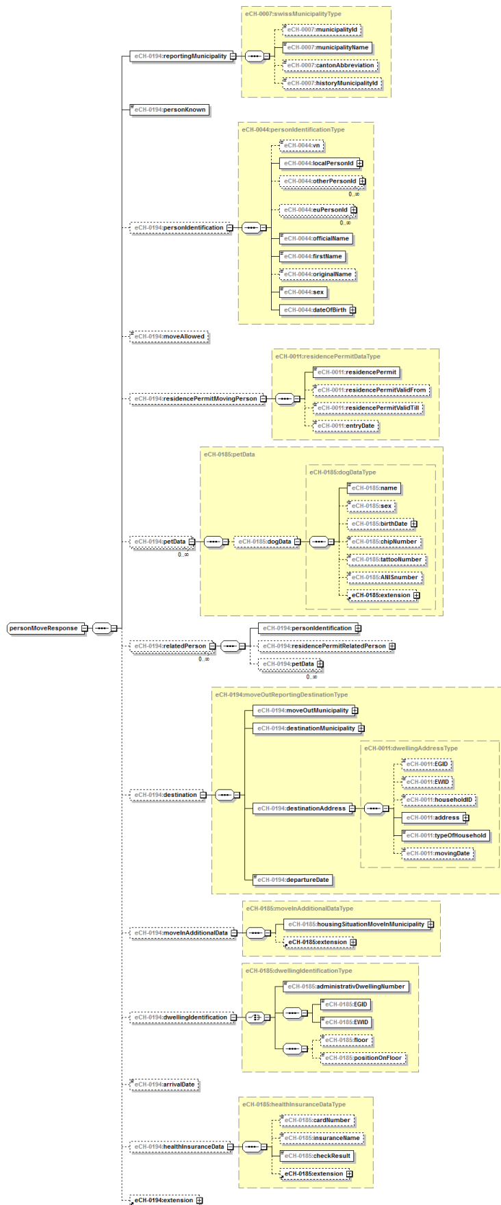
Abbildung 7: personMoveResponse
