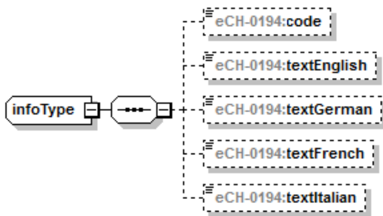
Abbildung 16: infoType
