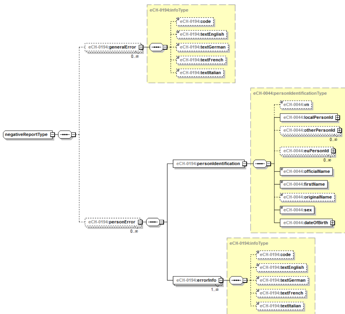
Abbildung 15: negativeReport
