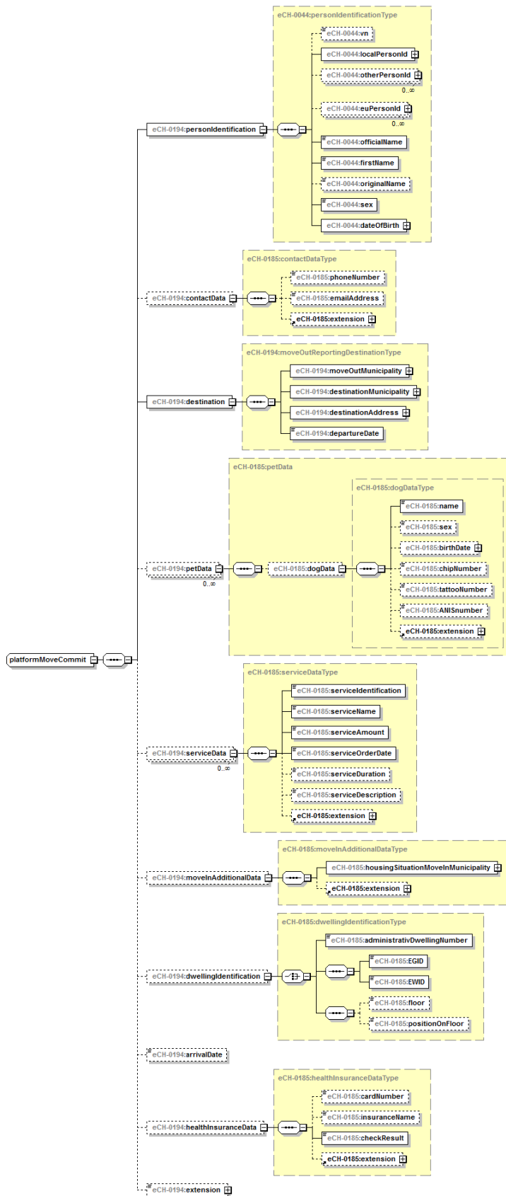
Abbildung 12: platformMoveCommit
